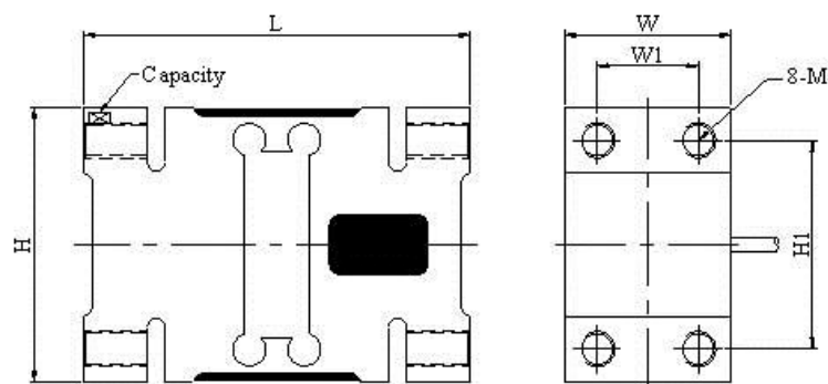
主视 (Front View)
